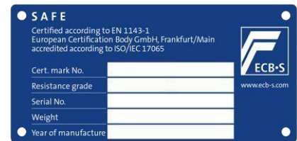
Beispiel Typenschild ECB-S-Tresore
